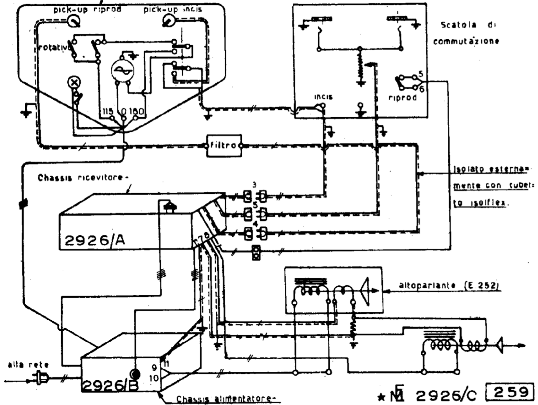
Il cablaggio del mod. « 2940 » radiofonografo e incisore.
